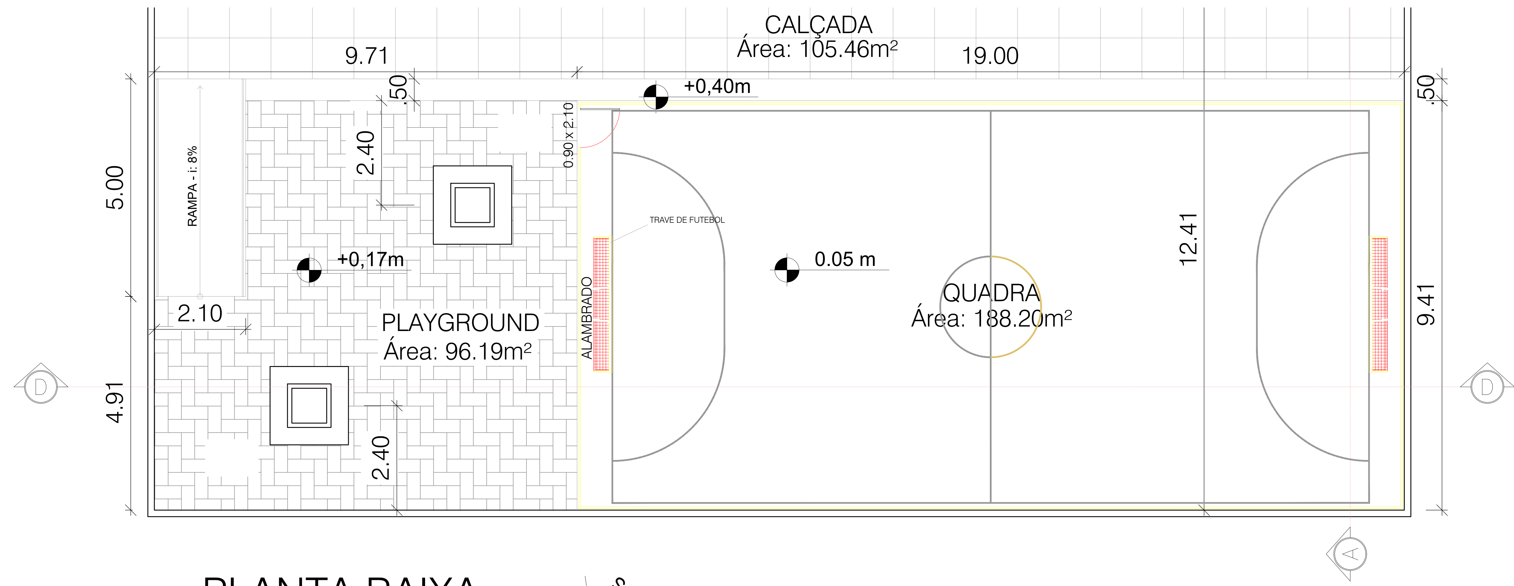
PLANTA BAIXA ESCALA 1:50
